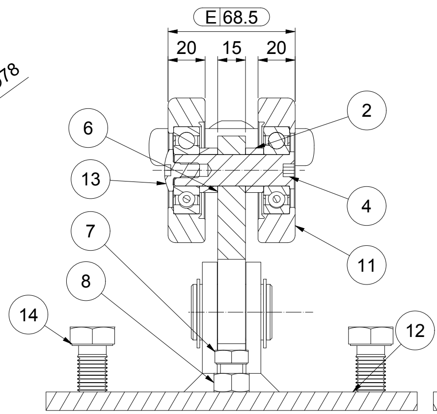
A-A ( 1 : 2 )
