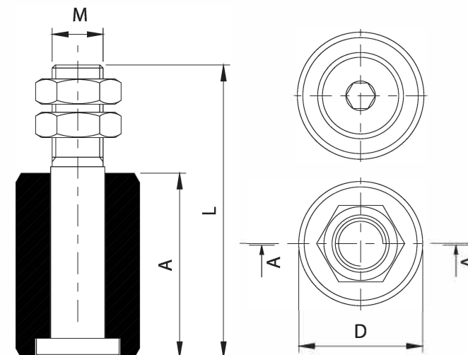
SEZ A-A
